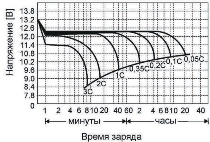
Разрядная характеристика АКБ
