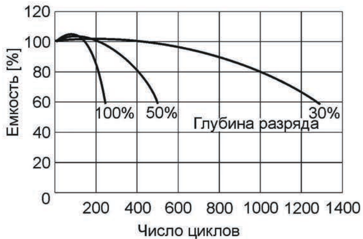
Срок службы АКБ в циклах
